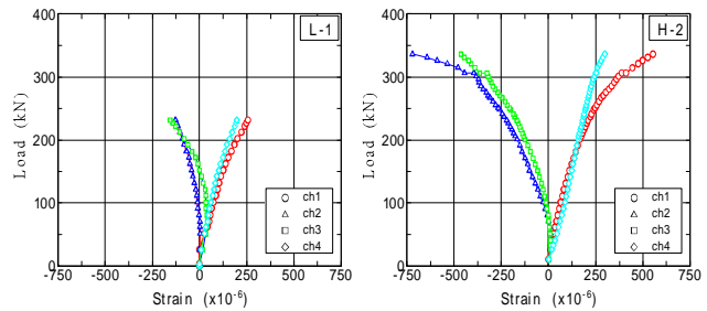
図-3 荷重-ひずみ曲線
