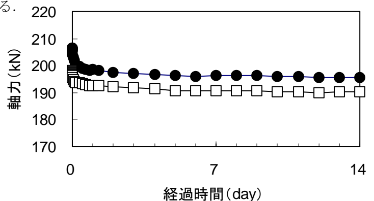
図-3. 軸力リラクゼーション試験結果
