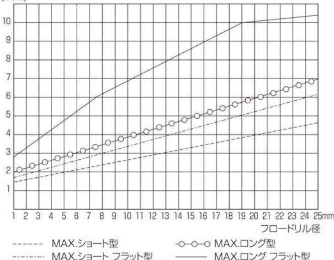
板厚 (mm.) 板厚によるフロードリル選定表
